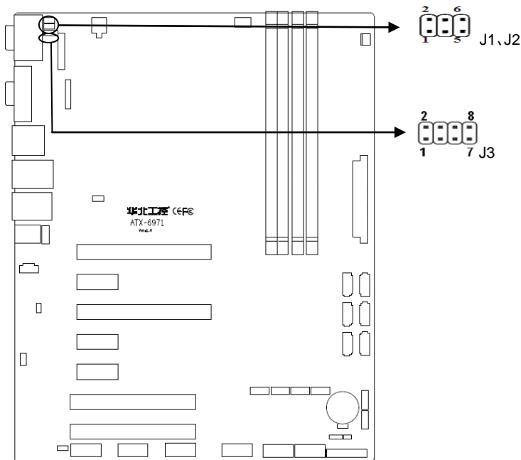
J1、J2、J3:
