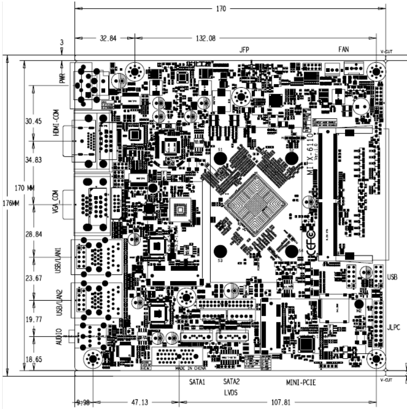
MITX-6110 接口位置和尺寸图
