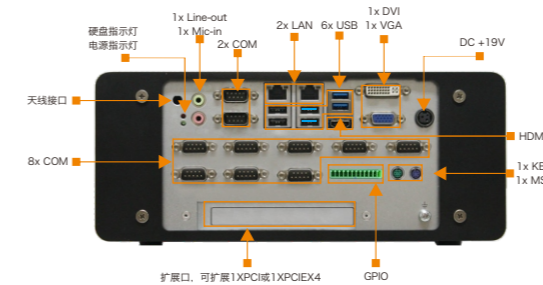
BIS-6910E接口
